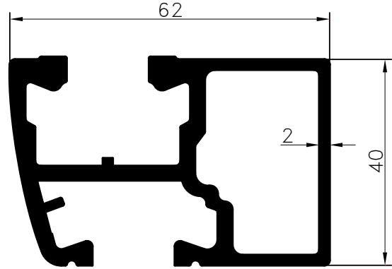
Pr.No: 9314 1,722 kg/m ÖZEL/PRIVATE
