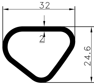
Pr.No: 8090 0,451 kg/m
