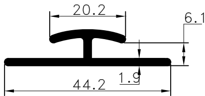
Pr.No: 9196 0,366 kg/m
