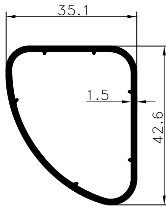
Pr.No: 8610 0,525 kg/m
