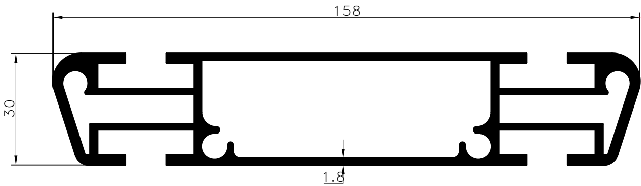
Pr.No: 9315 2,877 kg/m ÖZEL/PRIVATE
