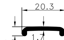
Pr.No: 9197 0,112 kg/m
