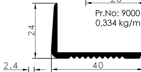
Pr.No: 9147 0,336 kg/m
