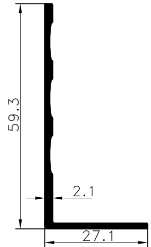
Pr.No: 9194 0,372 kg/m
