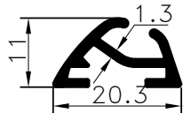
Pr.No: 8948 0,179 kg/m ÖZEL/PRIVATE
