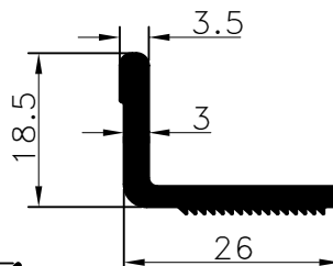
Pr.No: 9000 0,334 kg/m
