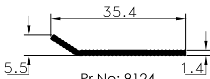
Pr.No: 9124 0,127 kg/m
