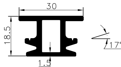
Pr.No: 9363 0,514 kg/m ÖZEL/PRIVATE
