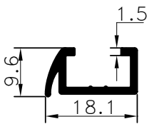
Pr.No: 8946 0,148 kg/m ÖZEL/PRIVATE
