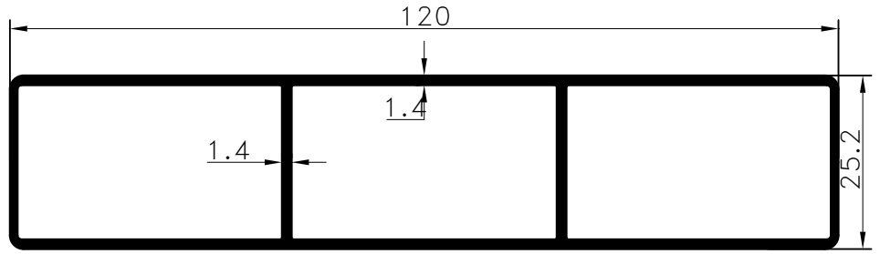
Pr.No: 8972 1,206 kg/m
