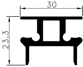
Pr.No: 9313 0,585 kg/m ÖZEL/PRIVATE
