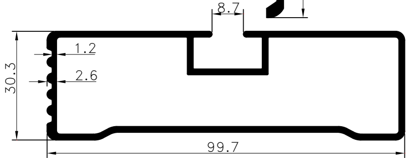
Pr.No: 8948 0,179 kg/m ÖZEL/PRIVATE
