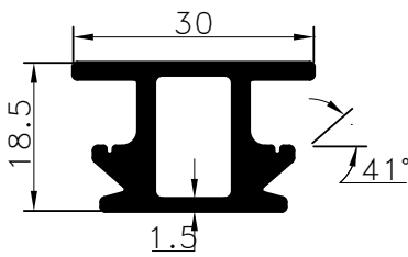
Pr.No: 9362 0,542 kg/m ÖZEL/PRIVATE
