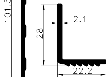
Pr.No: 9233 0,266 kg/m
