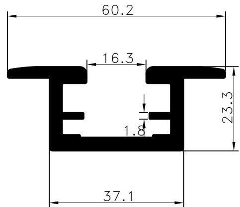
Pr.No: 9404 1,190 kg/m ÖZEL/PRIVATE
