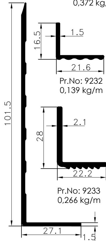
Pr.No: 8765 0,574 kg/m
