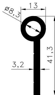
Pr.No: 9477 0,460 kg/m ÖZEL/PRIVATE
