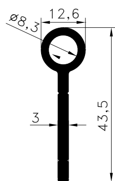
Pr.No: 9478 0,442 kg/m ÖZEL/PRIVATE
