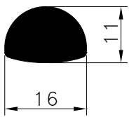
Pr.No: 8073 0,382 kg/m
