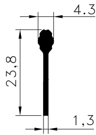
Pr.No: 8081 0,119 kg/m
