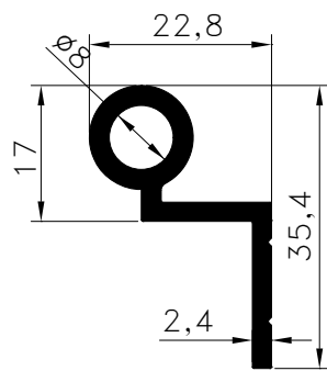
Pr.No: 8115 0,460 kg/m
