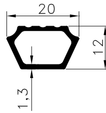
Pr.No: 8077 0,173 kg/m
