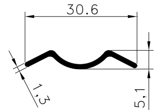
Pr.No: 8078 0,122 kg/m
