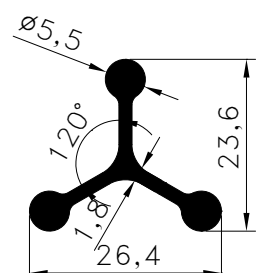
Pr.No: 8604 0,339 kg/m
