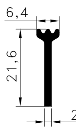
Pr.No: 8105 0,141 kg/m
