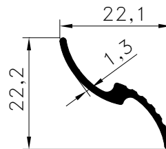
Pr.No: 8082 0,136 kg/m
