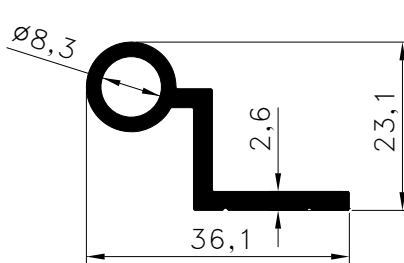
Pr.No: 9479 0,442 kg/m ÖZEL/PRIVATE
