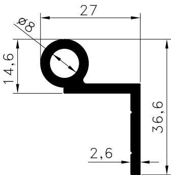
Pr.No: 8114 0,519 kg/m
