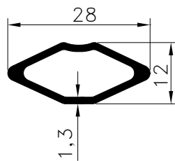
Pr.No: 8076 0,221 kg/m
