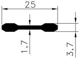
Pr.No: 8573 0,176 kg/m
