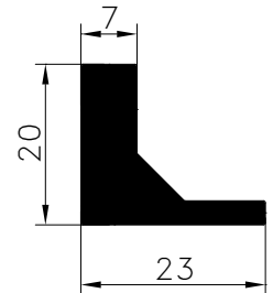
Pr.No: 9433 0,530 kg/m
