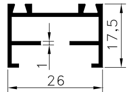
Pr.No: 8104 0,243 kg/m
