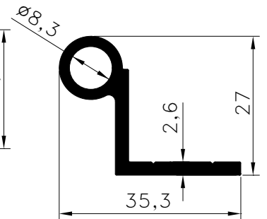
Pr.No: 9480 0,442 kg/m ÖZEL/PRIVATE
