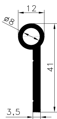
Pr.No: 8116 0,450 kg/m
