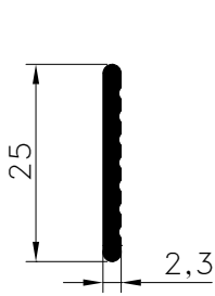
Pr.No: 8083 0,147 kg/m
