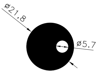
Pr.No: 8594 0,943 kg/m
