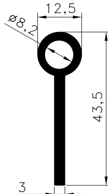
Pr.No: 8618 0,444 kg/m
