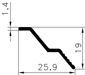
Pr.No: 8079 0,124 kg/m
