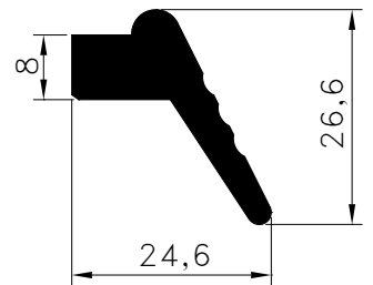
Pr.No: 8068 0,556 kg/m
