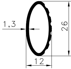
Pr.No: 8075 0,191 kg/m
