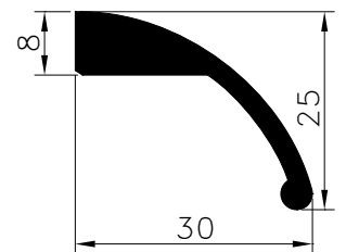
Pr.No: 8072 0,450 kg/m
