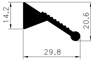
Pr.No: 8071 0,459 kg/m
