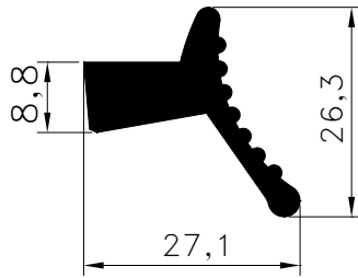
Pr.No: 8070 0,556 kg/m
