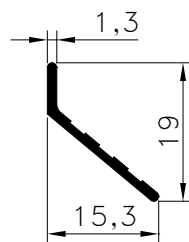
Pr.No: 8080 0,085 kg/m
