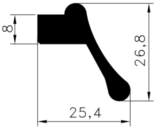
Pr.No: 8069 0,535 kg/m
