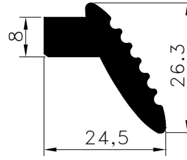
Pr.No: 8067 0,614 kg/m
