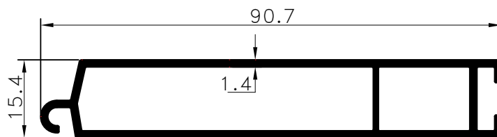
Pr.No: 9138 0,828 kg/m
