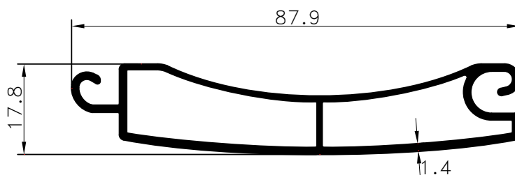
Pr.No: 9139 0,779 kg/m
