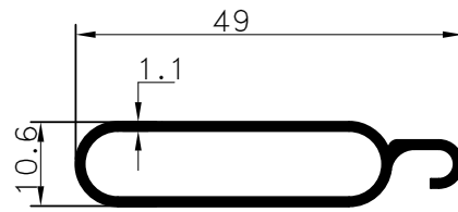
Pr.No: 8012 0,312 kg/m
