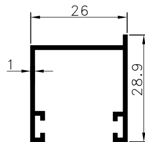
Pr.No: 8011 0,257 kg/m
