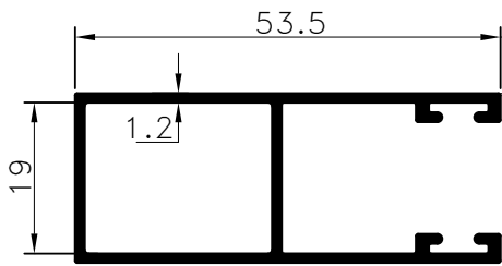
Pr.No: 8694 0,520 kg/m
