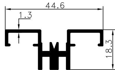
Pr.No: 8614 0,482 kg/m ÖZEL/PRIVATE
