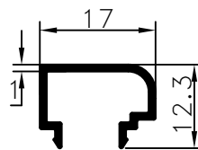
Pr.No: 8616 0,120 kg/m ÖZEL/PRIVATE
