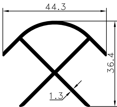
Pr.No: 8596 0,472 kg/m ÖZEL/PRIVATE
