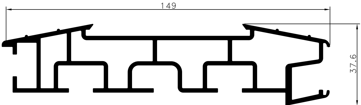
Pr.No: 8677 2,878 kg/m ÖZEL/PRIVATE
