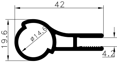
Pr.No: 8630 0,472 kg/m ÖZEL/PRIVATE
