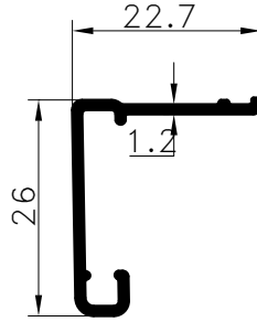
Pr.No: 8862 0,190 kg/m
