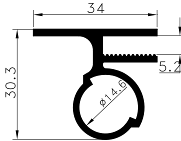
Pr.No: 8008 0,552 kg/m
