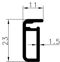
Pr.No: 8511 0,256 kg/m ÖZEL/PRIVATE
