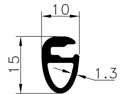
Pr.No: 9356 0,273 kg/m
