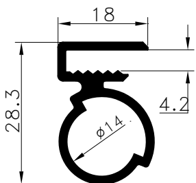
Pr.No: 9115 0,406 kg/m
