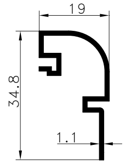
Pr.No: 8813 0,238kg/m ÖZEL/PRIVATE
