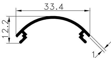
Pr.No: 8130 0,141 kg/m
