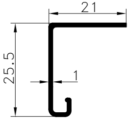
Pr.No: 8580 0,145 kg/m ÖZEL/PRIVATE
