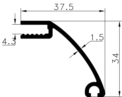
Pr.No: 8007 0,582 kg/m
