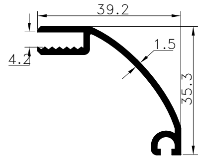
Pr.No: 8137 0,346 kg/m
