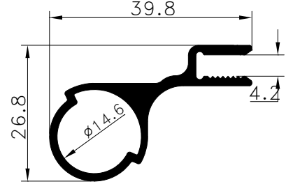
Pr.No: 9214 0,478 kg/m ÖZEL/PRIVATE
