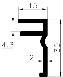
Pr.No: 8597 0,313 kg/m
