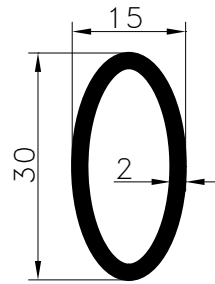
Pr.No: 8707 0,360 kg/m
