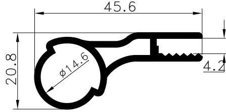
Pr.No: 8696 0,503 kg/m ÖZEL/PRIVATE
