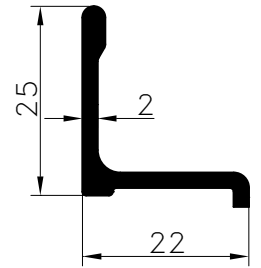
Pr.No: 8552 0,280 kg/m
