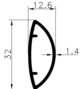
Pr.No: 9356 0,273 kg/m
