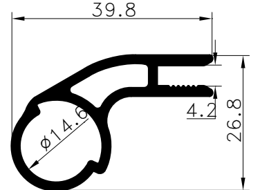
Pr.No: 9357 0,517 kg/m
