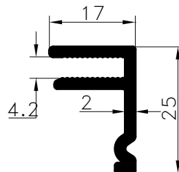
Pr.No: 9240 0,308 kg/m
