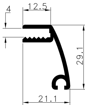
Pr.No: 9382 0,286 kg/m
