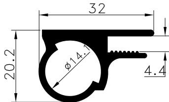
Pr.No: 8542 0,497 kg/m
