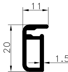
Pr.No: 8096 0,233 kg/m ÖZEL/PRIVATE
