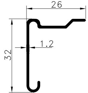
Pr.No: 8805 0,217 kg/m ÖZEL/PRIVATE
