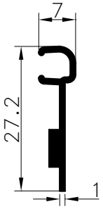
Pr.No: 8619 0,141 kg/m
