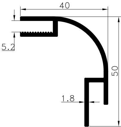
Pr.No: 8007 0,582 kg/m
