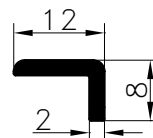
Pr.No: 9484 0,095 kg/m ÖZEL/PRIVATE
