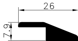
Pr.No: 9483 0,244 kg/m ÖZEL/PRIVATE
