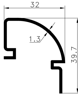
Pr.No: 8583 0,347 kg/m ÖZEL/PRIVATE
