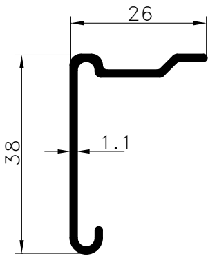
Pr.No: 9215 0,218 kg/m
