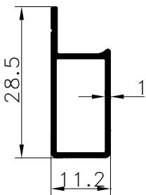
Pr.No: 8772 0,187 kg/m
