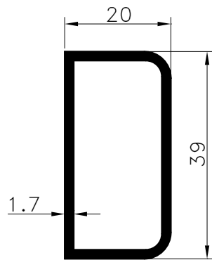
Pr.No: 8005 0,492 kg/m
