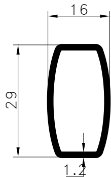
Pr.No: 9267 0,253 kg/m
