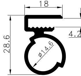
Pr.No: 8138 0,410 kg/m
