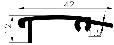
Pr.No: 8625 0,279 kg/m ÖZEL/PRIVATE
