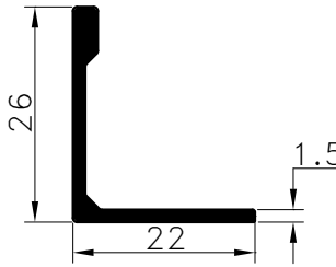
Pr.No: 8650 0,216 kg/m
