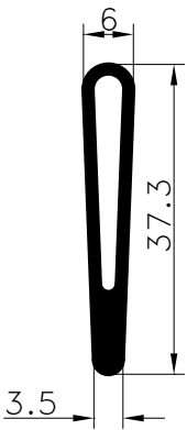
Pr.No: 9252 0,266 kg/m
