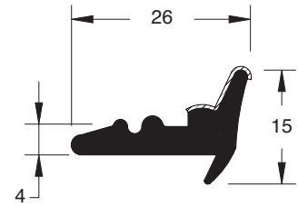
0690 EPDM
