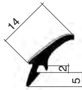
0001 (mm. 2120) EPDM
