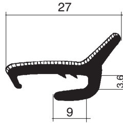
4006 EPDM
